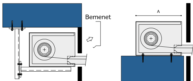
Mennyezeti rögzítés
